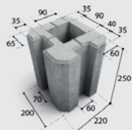
PZ25 ECO NAROŻNY
