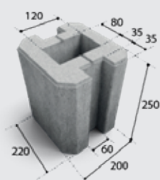
PZ25 ECO PRZELOTOWY
